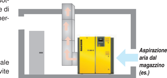
Fig. 3: Aerazione forzata con aria di espulsione canalizzata, per macchine superiori a 11 kW
